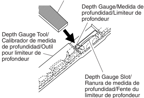
Figure 21 - Depth Gauge Tool On Chain Figura 21 - Calibrador de medida de profundidad en la cadena
